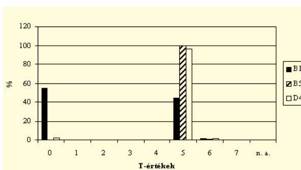
2. ábra A Zólyomi-féle T-értékek megoszlása a vizsgált Á-NÉR típusokban (jelölést lásd 1. ábra).
