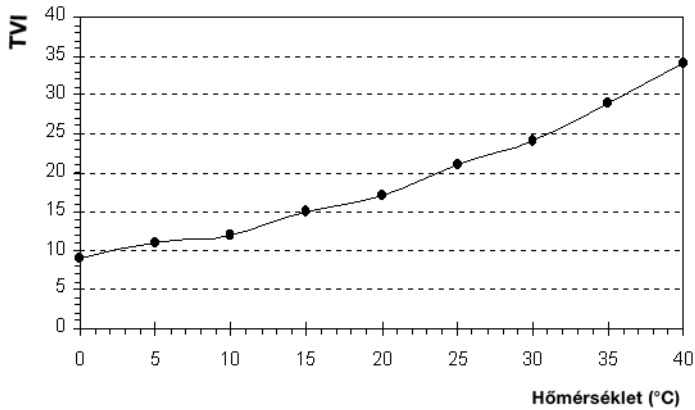
3. ábra A TVI (tűzveszélyességi index) változása a hőmérséklettel, bármely állománykor esetén (mivel a TVI független az éghető anyag mennyiségétől). Relatív humiditás= 30%, szélsebesség= 30 km/h, szárazsági faktor= 10, lejtőszög= 30°.
