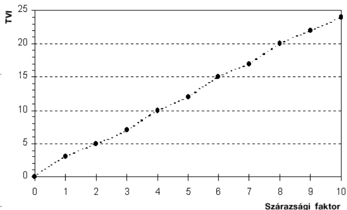
6. ábra A TVI (tűzveszélyességi index) változása a szárazsági faktoral, bármely állománykor esetén (mivel a TVI független az éghető anyag mennyiségétől). Hőmérséklet= 30 °C, relatív humiditás= 30%, szélsebesség= 30 km/h, lejtőszög= 30°.
