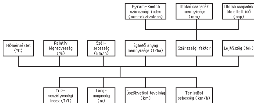
1. ábra A McArthur-féle tűzveszélyességi modell felépítése. Figure 1. Schematic diagram of the McArthur's model.
