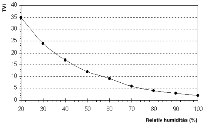
4. ábra A TVI (tűzveszélyességi index) változása a relatív páratartalommal, bármely állománykor esetén (mivel a TVI független az éghető anyag mennyiségétől). Hőmérséklet= 30 °C, szélsebesség= 30 km/h, szárazsági faktor= 10, lejtőszög= 30°.
