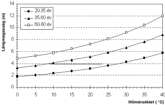
7. ábra A lángmagasság változása a hőmérséklettel, három korcsoport esetén. Relatív humiditás= 30%, szélesebbég= 30 km/h, szárazsági faktor= 10, lejtőszög= 30°, éghető anyag mennyisége a korcsoportokban: 20-35 év= 10574 kg/ha; 35-60 év= 14024 kg/ha; 60-80 év= 18564 kg/ha.
