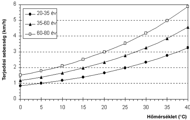
15. ábra A tűz terjedési sebességének változása a hőmérséklettel, három korcsoport esetén. Relatív humiditás= 30%, szélsebesség= 30 km/h, szárazsági faktor= 10, lejtőszög= 30°.
