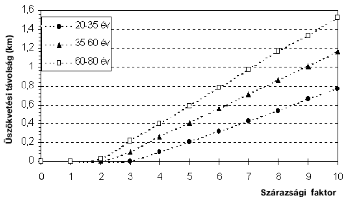
14. ábra Az üszökvetési távolság változása a szárazsági faktoral, három korcsoport esetén. Hőmérséklet= 30 °C, relatív humiditás= 30%, szélsebesség= 30 km/h, lejtőszög= 30°.
