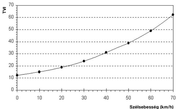
5. ábra A TVI (tűzveszélyességi index) változása a szélsebességgel, bármely állománykor esetén (mivel a TVI független az éghető anyag mennyiségétől). Hőmérséklet= 30 °C, relatív humiditás= 30%, szárazsági faktor= 10, lejtőszög= 30°.
