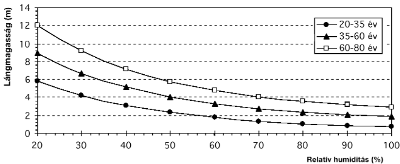
8. ábra A lángmagasság változása a relatív páratartalommal, három korcsoport esetén. Hőmérséklet= 30 °C, szélesebbég= 30 km/h, szárazsági faktor= 10, lejtőszög= 30°. A figyelembe vett éghető anyag mennyiségek azonosak a 7. ábránál megadottakkal. Figure 8. Changes of the flame height with the relative air humidity in the three stand age classes. Constant parameters: temperature= 30 °C, wind speed= 30 km/h, drought factor value= 10, slope angle= 30°. See Fig. 7 for the amounts of fuel considered in the three stand age classes.
