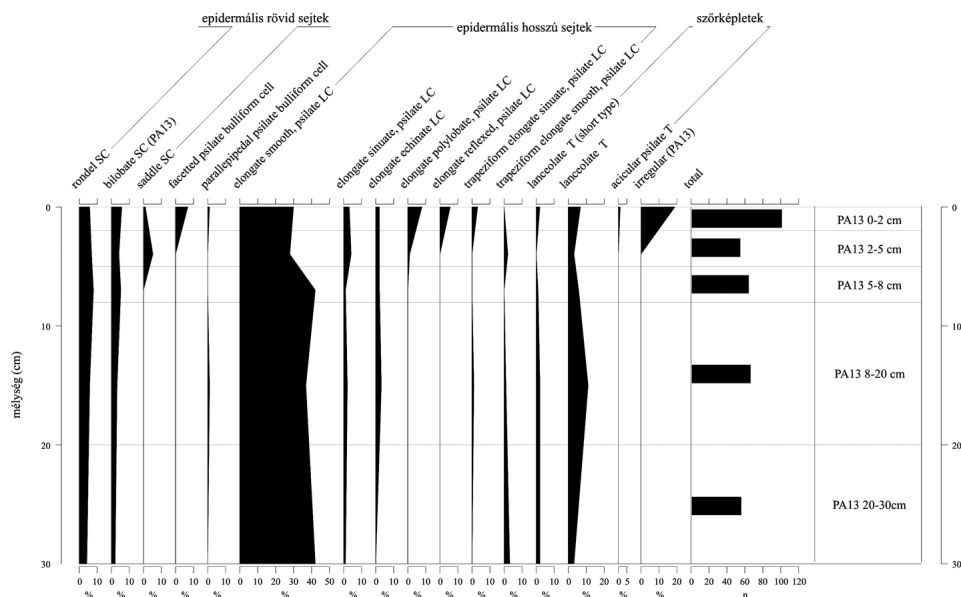
16. ábra A PA13 erősen savanyú, nem podzolos barna erdőtalaj morfolópus-összetétele és fitoliteloszlási görbéje Figure 16. Vertical phytolith distribution and morphotype spectra of PA13 brown forest soil profile
