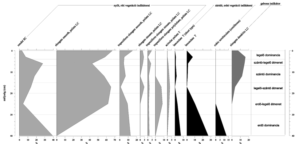
15. ábra A PA01 agyagbemosódásos barna erdőtalaj fitoliteloszlási görbéjére alapozott területhasználati rekonstrukció (PETŐ 2009 nyomán átszerkesztve) Figure 15. Reconstructed land use history based on the vertical phytolith distribution of the PA01 brown forest soil profile
