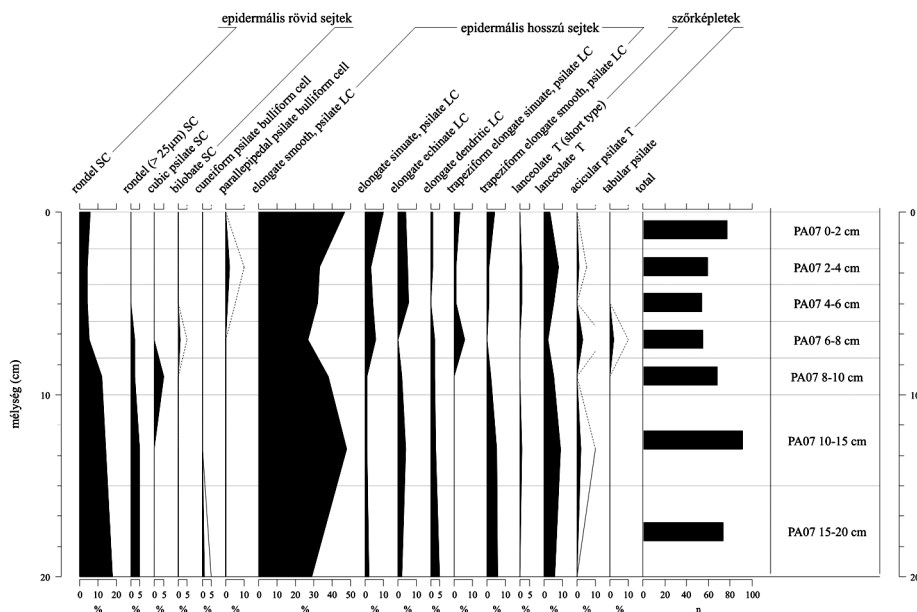
11. ábra A PA07 Ramann-féle barna erdőtalaj morfortípus-összetétele és fitoliteloszlási görbéje
