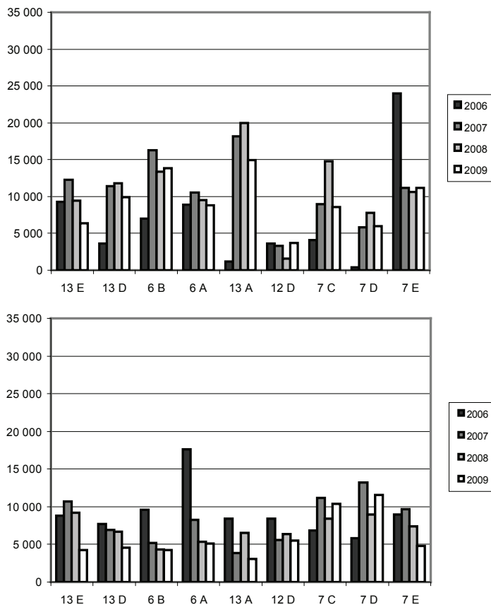
2. ábra Virágoskőrís és cser újulatok darabszámának évenkénti változása erdőrésztlenkénti átlagban Figure 2. Annual change of the number of stems per hectare in manna ash and turkey oak regenerations in stand average.
