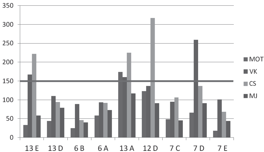
8. ábra Újulatok magassága erdőrészenként 2009-ben Figure 8. Height of regeneration by forest stands.
