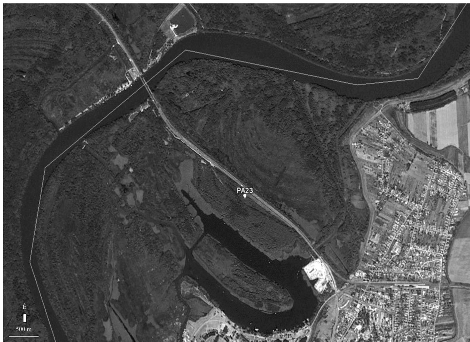
PA23 több rétegű humusos öntésalaj-szelvény elhelyezkedése (1:10 000 topográfiai térképszelvény; szerkesztett Google Earth szelvény)
