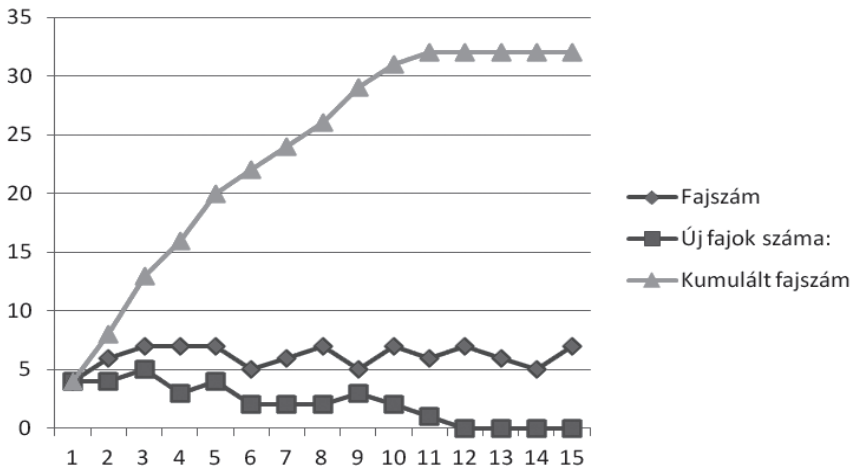
7. ábra A fajszám és a kumulált fajszám alakulása a bezárt kiskunhalasi hulladéklerakó területén végzett cönológiai felvételezés során Figure 7. Number of species and the cumulative number of species found during the phytosociological survey on the area of the closed landfill of Kiskunhalas
