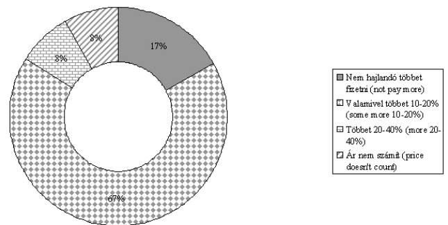
6. ábra Mennyivel hajlandóak többet fizetni az organikus édességekért? – How much are they willing to pay more for the organic sweets?
