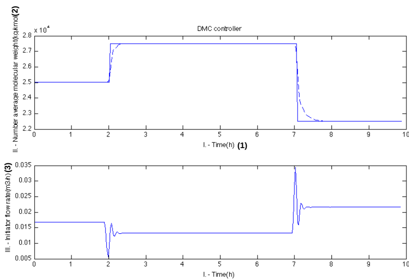
6. ábra: A DMC szabályozóval végzett szimuláció eredménye
