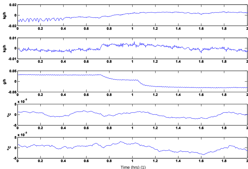
2. ábra: Példa egy C2 termékről C3 termékre történő termékváltásra (normalizált adatok, sorrendben: hidrogén betáplálás az 1. és 2. reaktorba, katalizátor betáplálása az 1. reaktorba, reaktor hőmérsékletek az 1. és 2. reaktorban).
