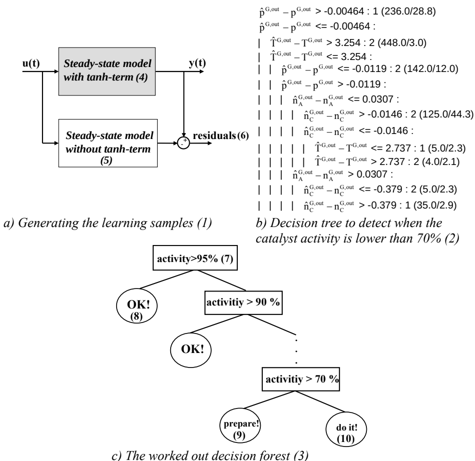
7. ábra: A katalizátor aktivitásának meghatározása döntési fa technikával
