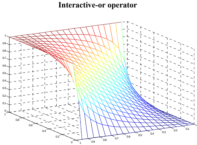
3. ábra: Az i-or operátor
