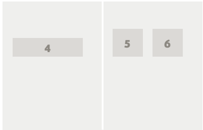
4. ábra/Fig. 4: Az FVT-k területén az új mesterséges felszín a vizsgált peródusokban / The new artificial surfaces during the examined periods in FUA areas. The size of the bubble indicates the share of the changed areas to the FUA area
