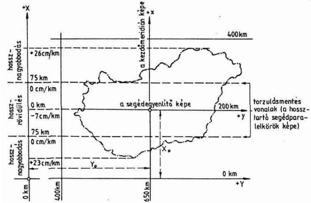
1. ábra/fig. 1: EOv hossztorzulása / Longitudinal distortion in the EOv system (FORRÁS/SOURCE: KRAUTER, ANDRÁS, GEODÉZIA, MŰEGYETEM KIADÓ, [BUDAPEST] 2002, p. 63.)
